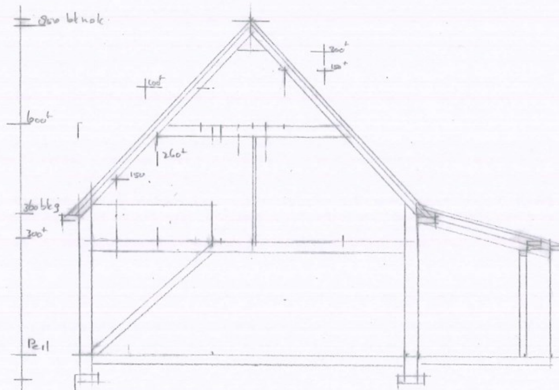
DOORSNEDE
