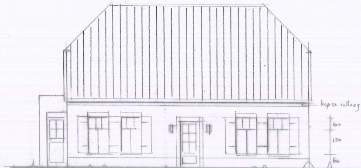
VOORGEVEL
