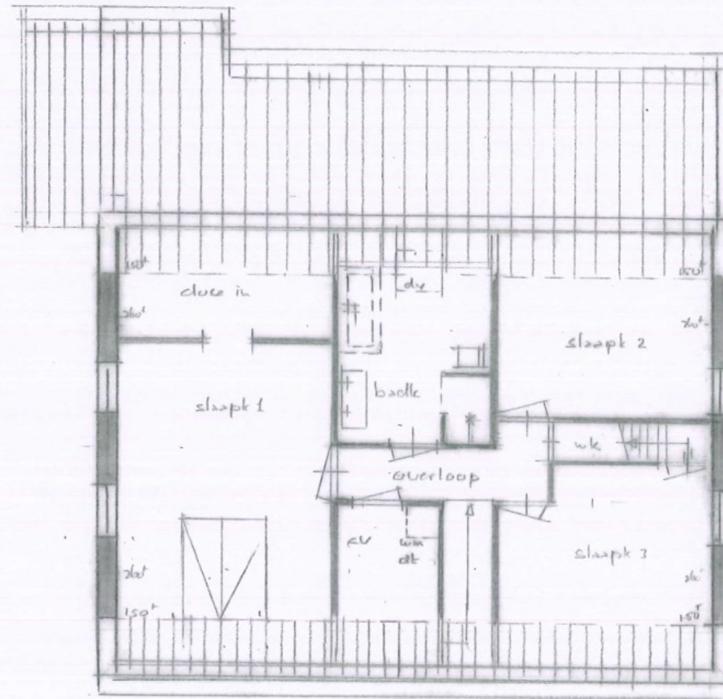
VERDIEPING 1
