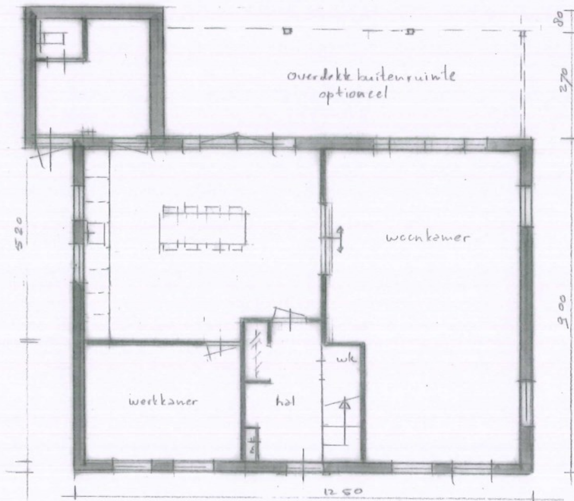
BEGANE GROND
