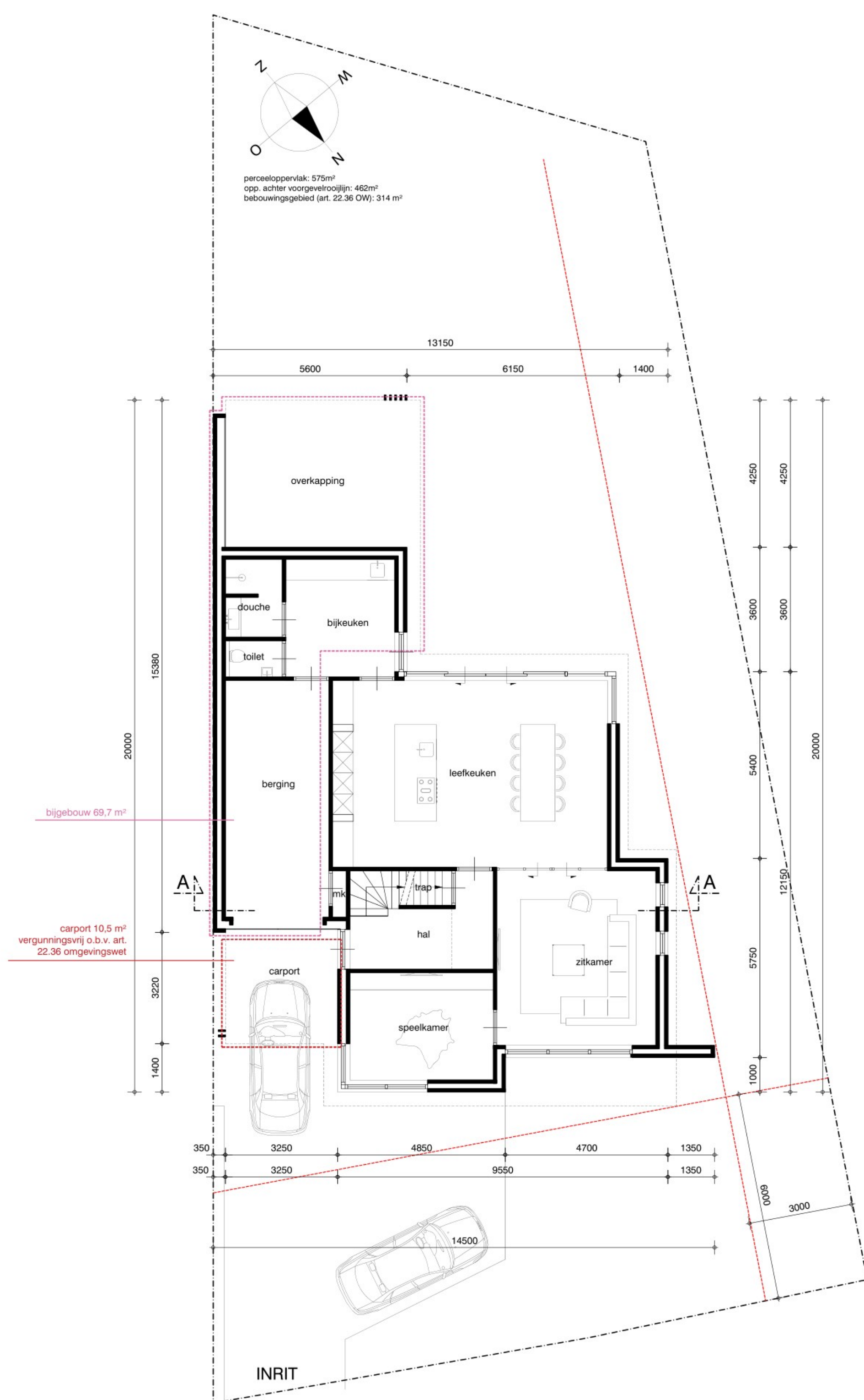
Begane Grond
