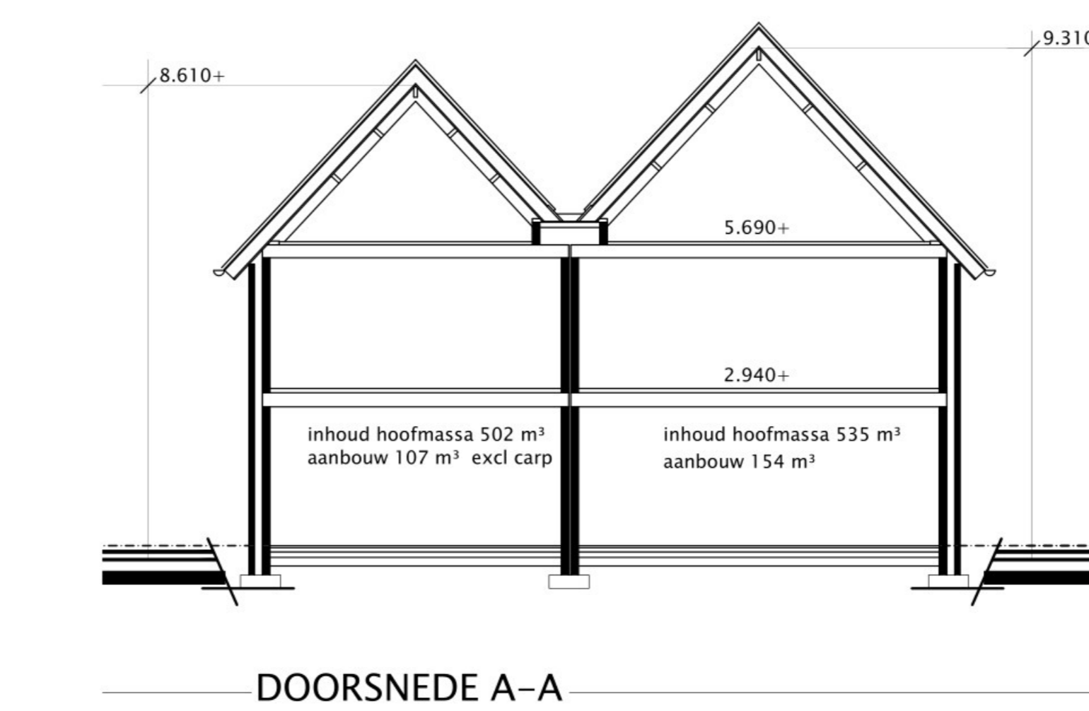
DOORSNEDE A-A
